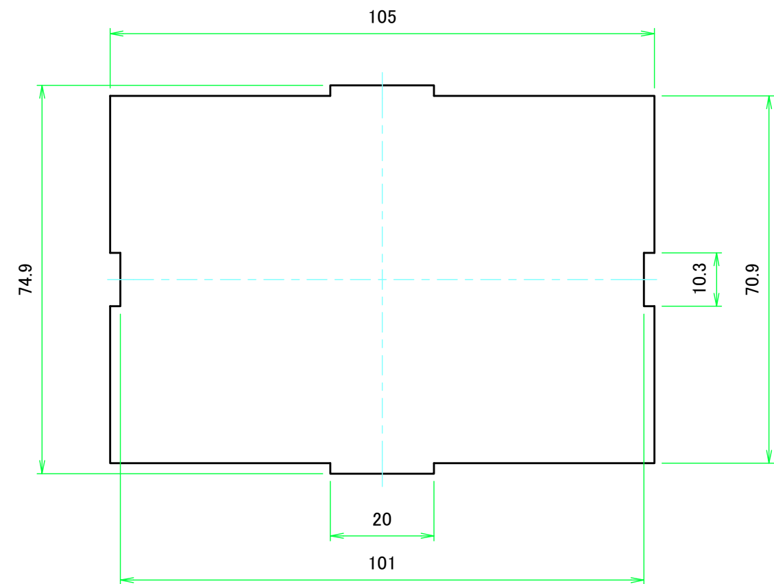
Wパネル1表面 / W Panel 1 Frontside
