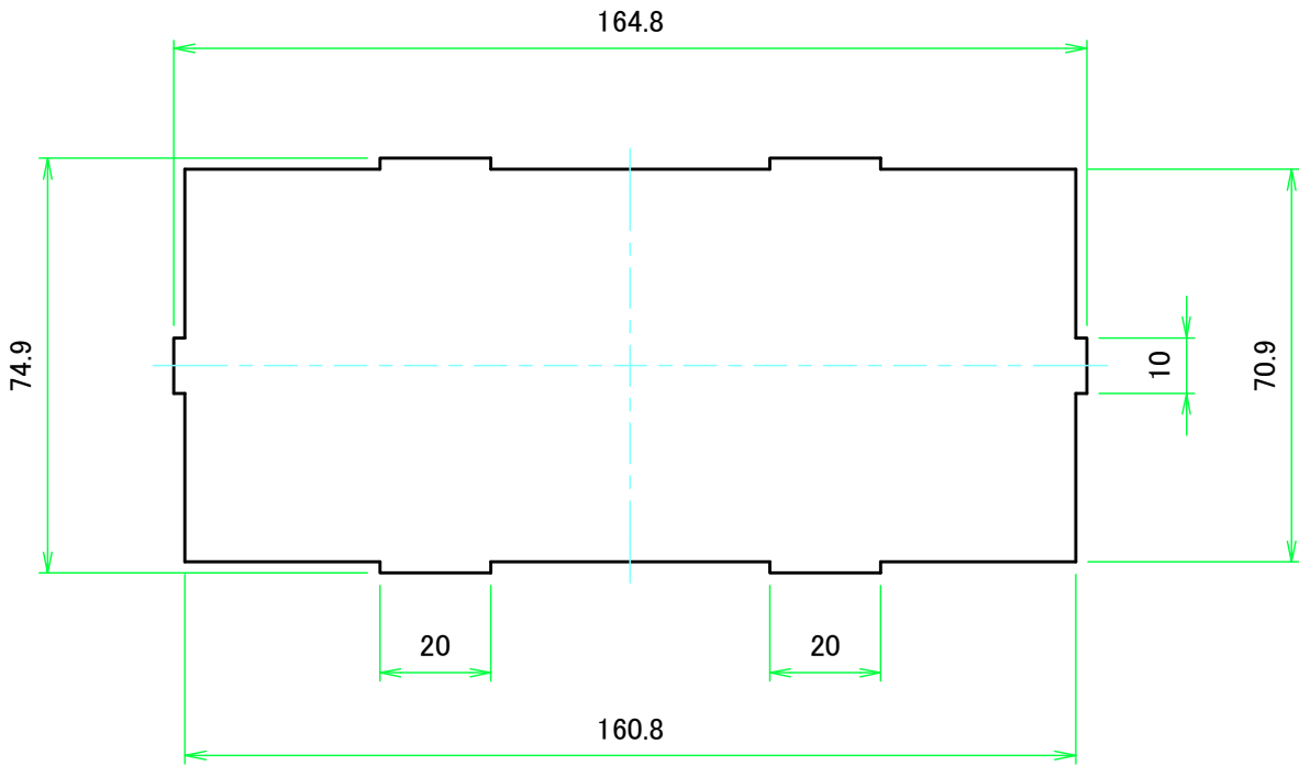
Dパネル1表面 / D Panel 1 Frontside
